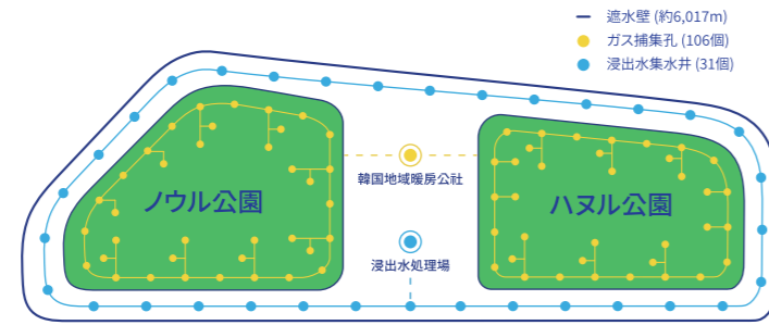
<浸出水処理施設及び埋立ガス処理施設の平面図>
