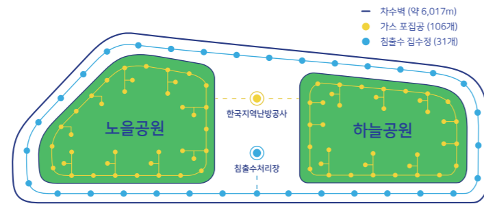
<침출수 및 매립가스 처리 평면도>
